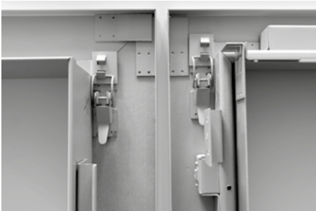
Zložené diely
