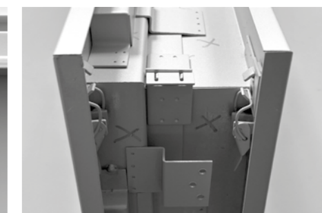
Kompletní zárubeň.
